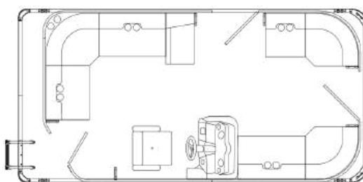
18' LE CR
